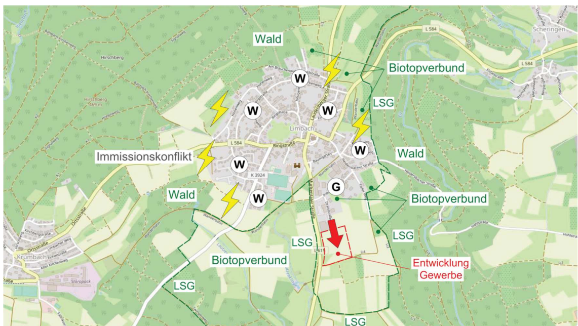
Abb. 7: Lageplan zur Prüfung von Standortalternativen (Quelle: Eigene Darstellung / Datengrundlage: www.openstreetmap.org )
